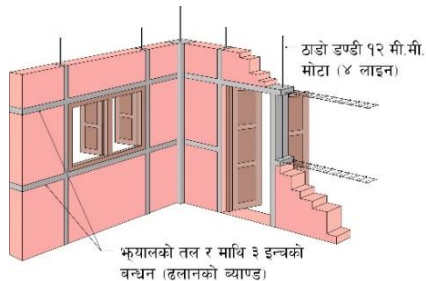
चित्र ४६: तेर्सो बन्धनको स्थान
