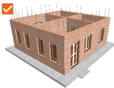
चित्र ४८: दुवै दिशामा दुई भन्दा बढि गारो भएका भवन
